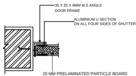
DETAIL AT A N.T.S.
