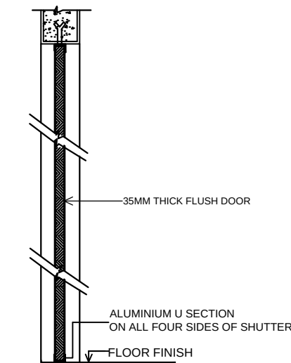
SECTION AT Y'-Y' N.T.S.
