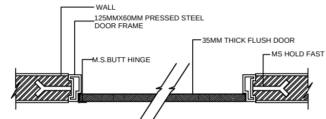
SECTION XX N.T.S.
