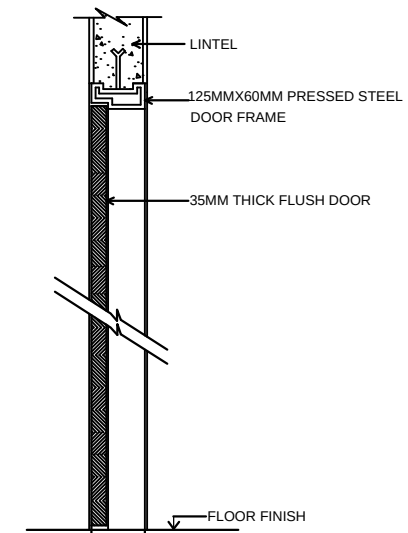
SECTION YY N.T.S.
