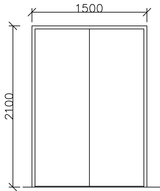
DOOR TYPE D
