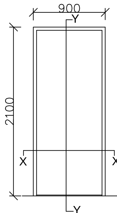
DOOR TYPE D2
