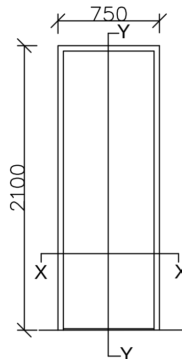
DOOR TYPE D3
